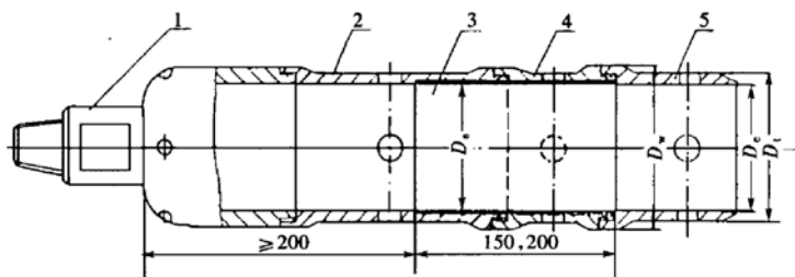
图 D—1 黄土薄壁取样器示意图
