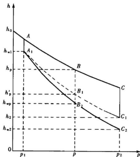
图 4.3.7 双线法压缩试验
